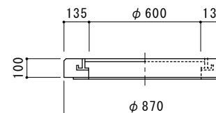
蓋受
