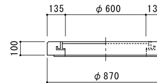
蓋受詳細
